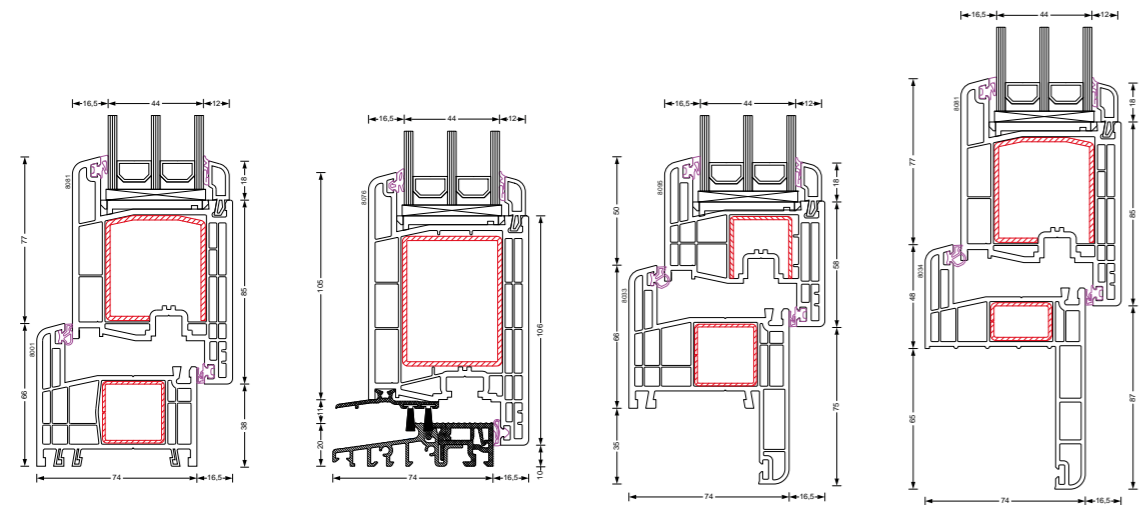
8001 - 8081 threshold - 8076 8033 - 8095 8034 - 8081
