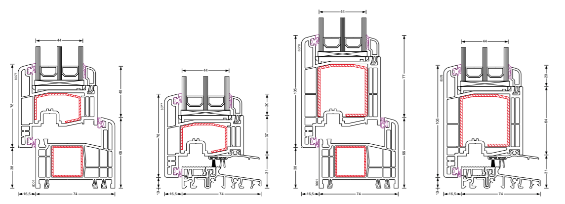
8001 - 8077 threshold - 8077 8001 - 8078 threshold - 8078
